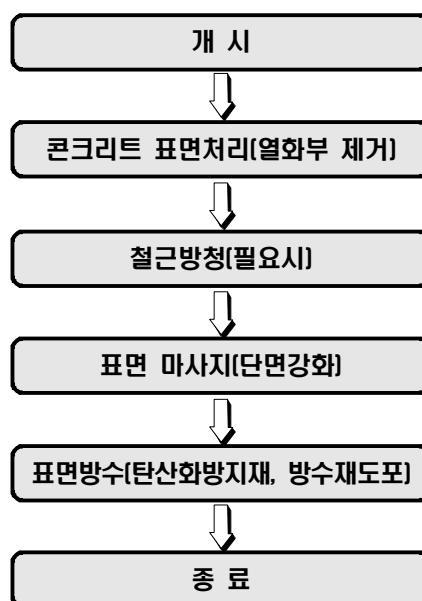
【그림 7.1】 표면처리공법 시공순서도
