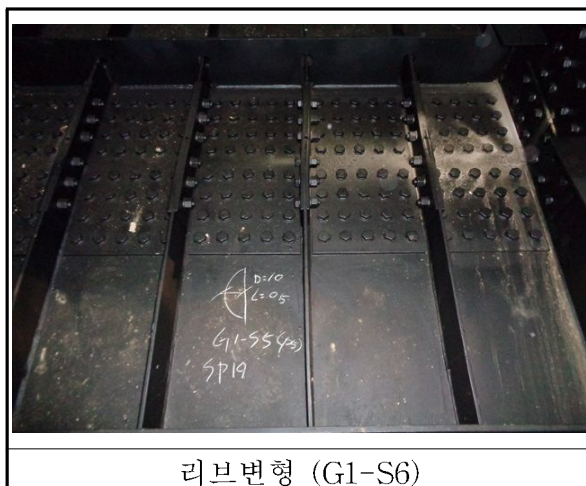
【그림 7.4】 리브 변형 현황
